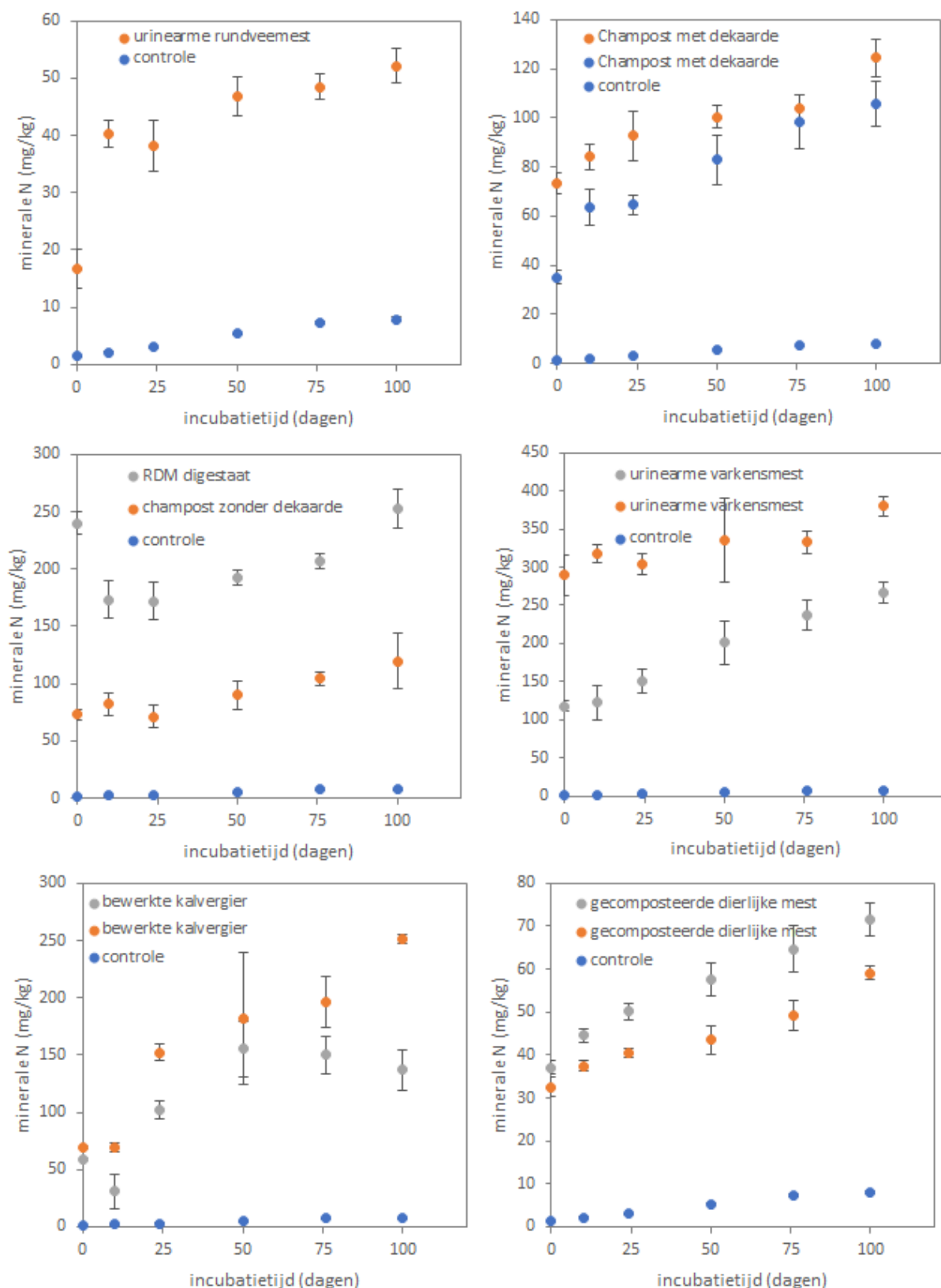
Figuur 3 Mineraal N (som van \text{NH}_4\text{-N} + \text{NO}_3\text{-N} + \text{NO}_2\text{-N} ) als functie van incubatietijd ( n=4 ). Het vochtgehalte van de grondmonsters was bij bemonstering 12 \pm 1,3\% . De toegevoegde hoeveelheid mest is steeds 20 gram vers monster per 200 gram verse grond. Om tot het constante vochtgehalte te komen, is rekening gehouden met het vocht van de mest. De verschillende kleuren (oranje/grijs) geven verschillende monsters aan. Om de data goed te laten zien, is de y-as niet hetzelfde bij alle figuren.
