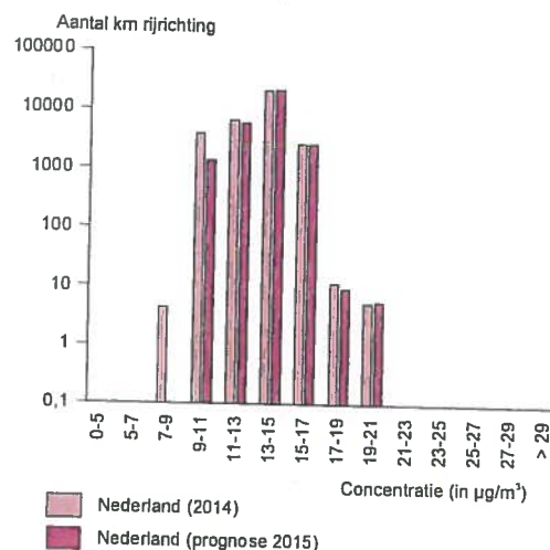
Concentratiehistogram PM_{2,5}
