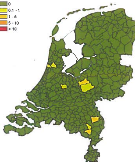
Figuur 24 PM 10 : Aantal overschrijdingen in 2020 getoetst aan de wettelijke grenswaarde rekening houdend met de zeezoutaf trek (links) en met bandbreedte (rechts). Exclusief overschrijdingen bij veehouderijen.
