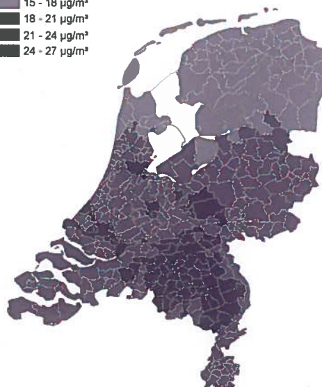
Figuur 25 Bevolkingsblootstelling aan NO 2 (links) en PM 10 (rechts) in 2020.
