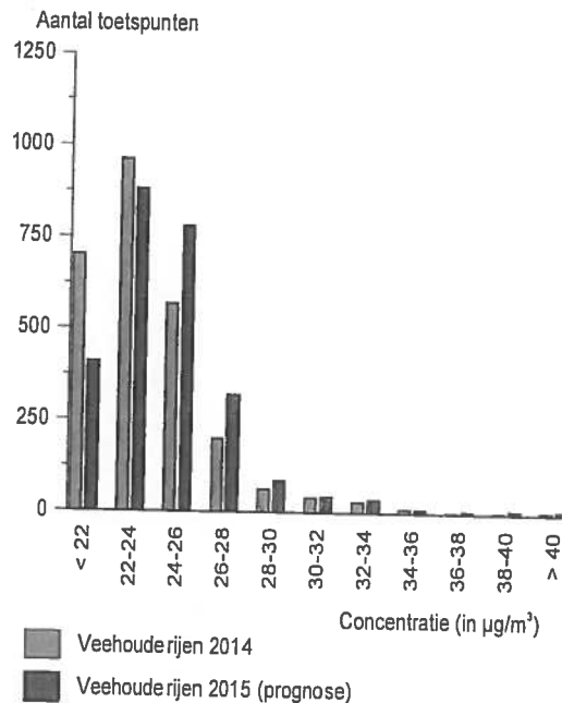
Totale jaargemiddelde fijn stof concentratie
